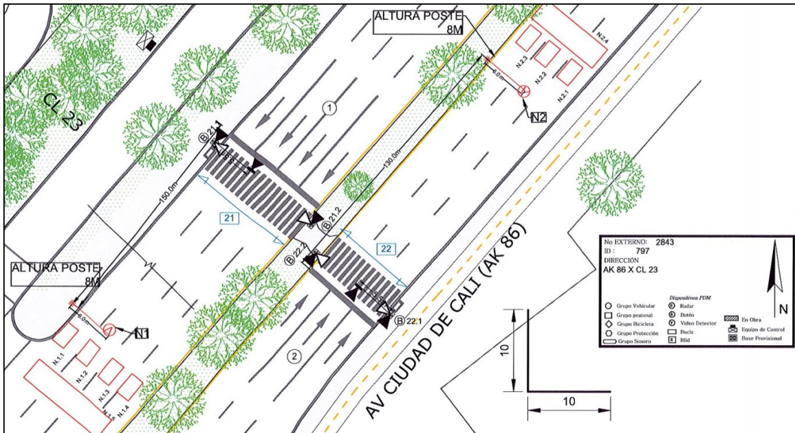
Figura 1. Esquema de la intersección Semaforizada AK 86 por CL 23.
