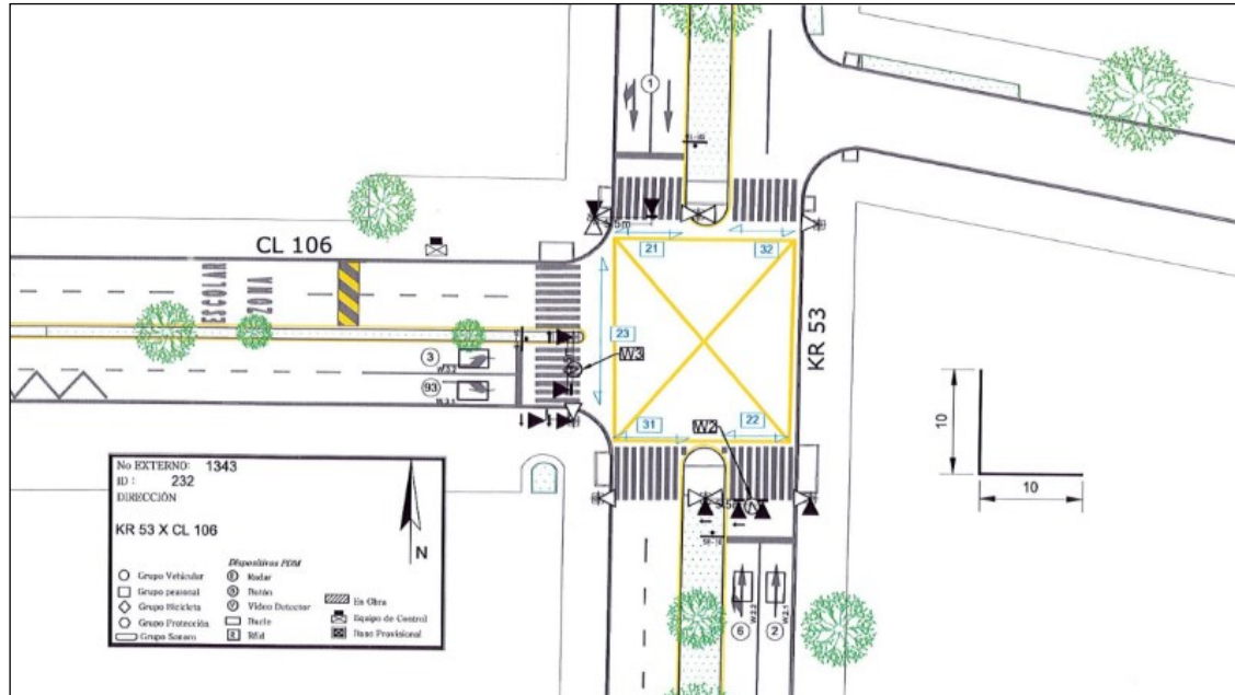
Figura 1. Esquema de la intersección Semaforzada Carrera 53 con Calle 106
