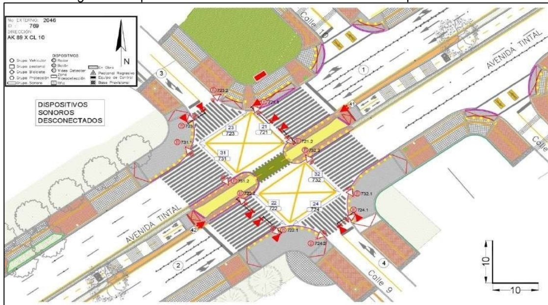
Figura 1. Esquema de la intersección Semaforizada AK 89 por CL 10.
