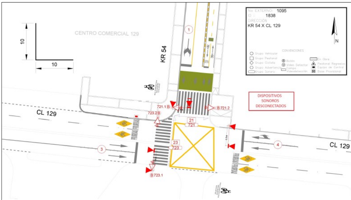
Figura 2. Esquema de la intersección KR 54 X CL 129
