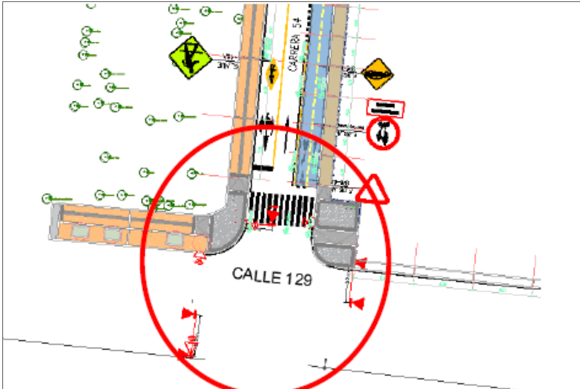
Figura 1. Diseño intersección KR 54 X CL 129
