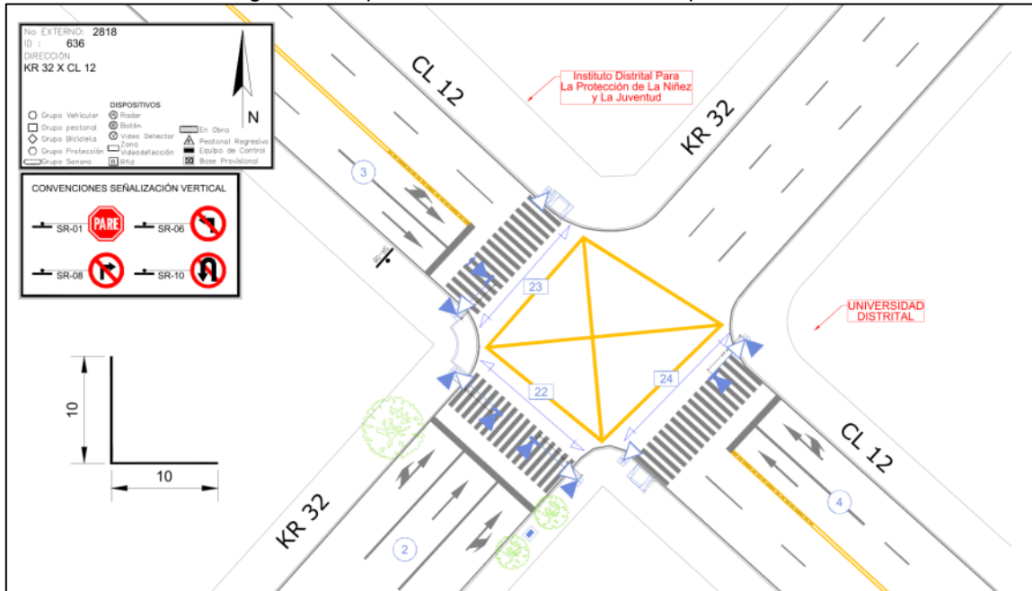
Figura 1. Esquema intersección carrera 32 por calle 12
