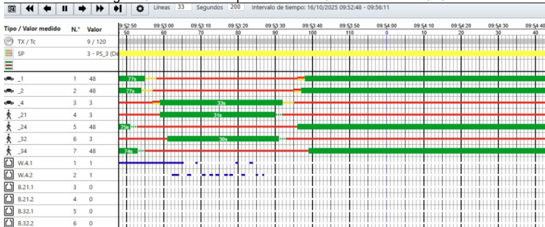
Figura 6. Revisión tiempos de verde 16 de octubre de 2025
