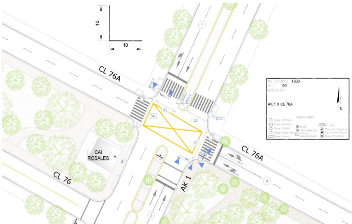
Figura 1. Esquema de la intersección AK 1 X CL 76A
